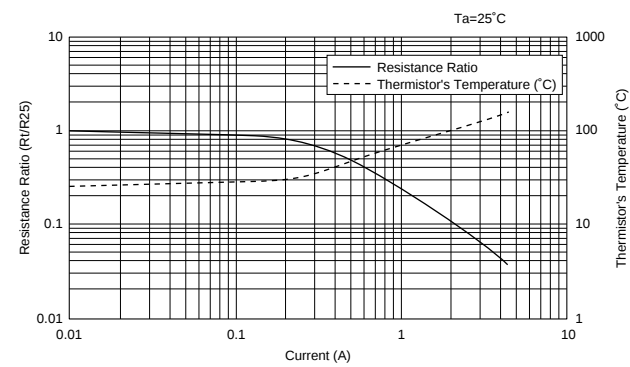
■ NTPDJ4R0L Type
