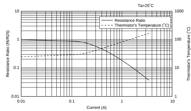
■ NTPDJ6R0L Type
