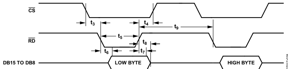
图30. 并行接口—字节操作模式的读取周期 ( \overline{\text{W}}/\text{B} = 1 , HBEN = 0)
