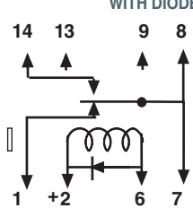
SPDT
