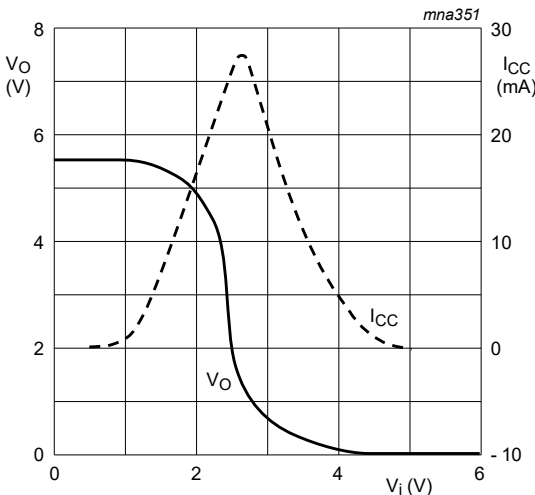
Fig. 8. V_{CC} = 5.5\text{ V} ; I_O = 0\text{ A}
