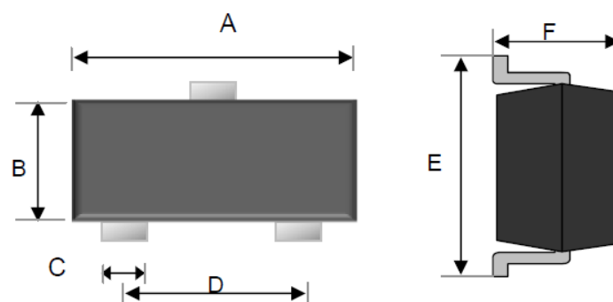
SOT-723
