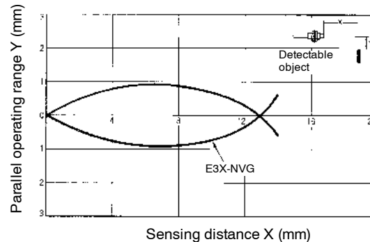
E32-D11L with E3X-NVG amplifier
