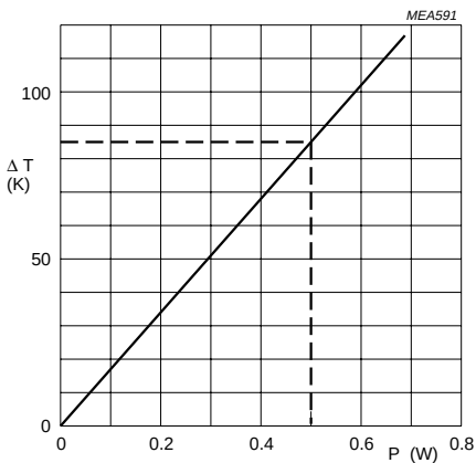
SFR16S 5033E
