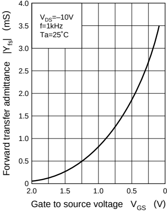
|Y_{fs}| - V_{GS}
