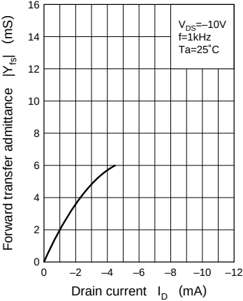
|Y_{fs}| - I_D
