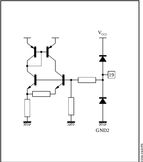
Figure 22 : Pin 19 - XRAY Input
