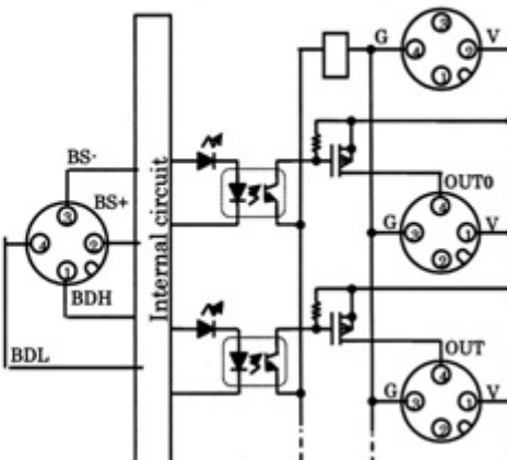
SRT2-OD0□CL(PNP)
