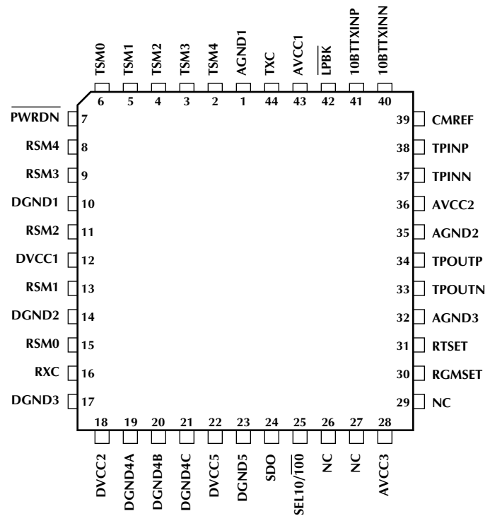
ML6694 44-Pin PLCC (Q44)
