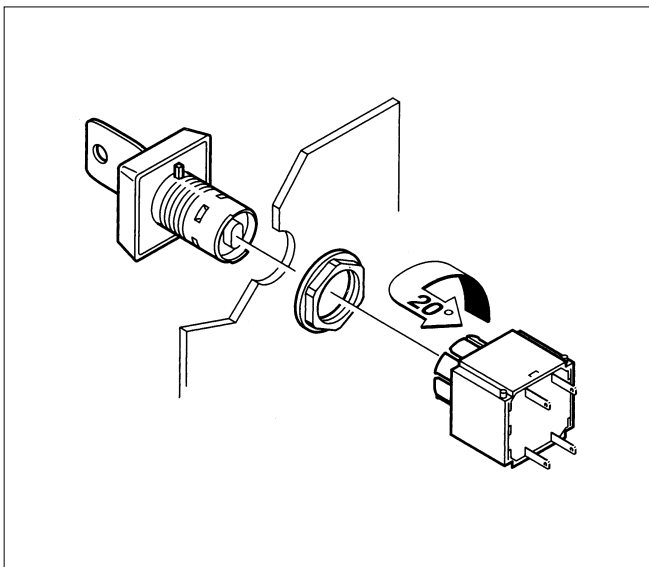
Montage/Demontage
