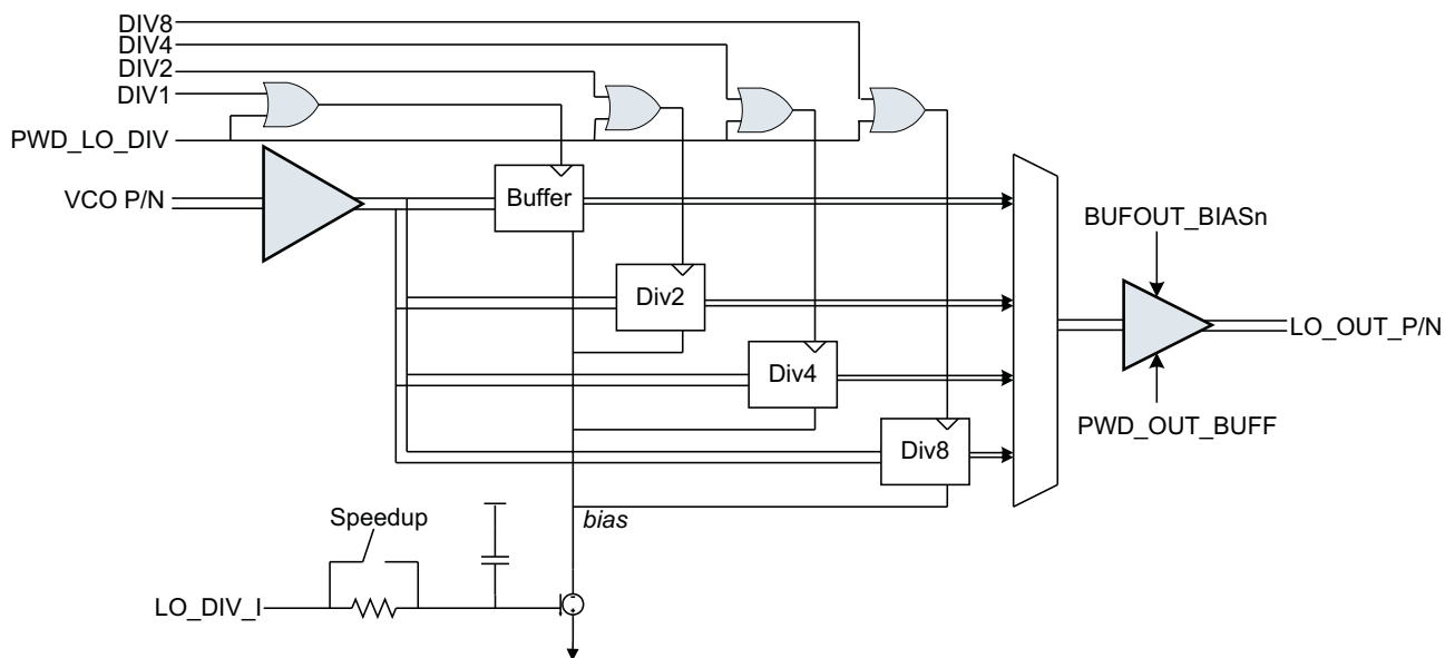
Figure 81. LO Divider
