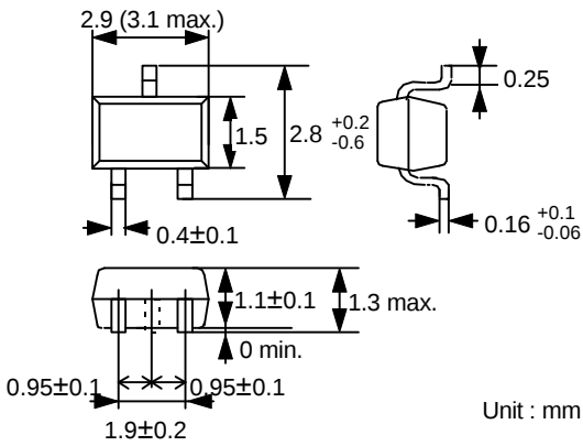
(2) SOT-23-3
