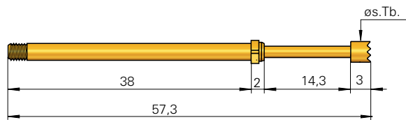
GKS-313 302 100 A xx02 M
