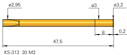
KS-313 30 M2
