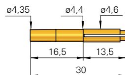
KS-VF5 030
