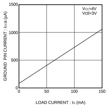
Fig.2 lcc vs. lo
