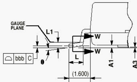
DETAIL Y
