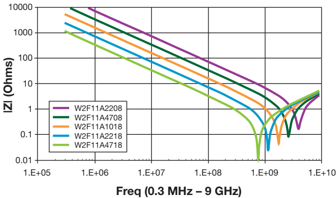
IMPEDANCE 0805 – 100V
