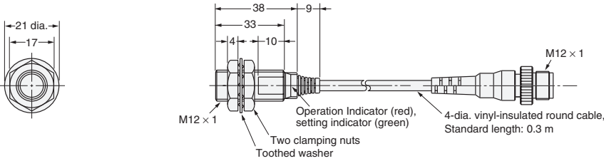
Fig. 30: E2E-X3D1-M1GJ E2E-X3D1-M1J-T
