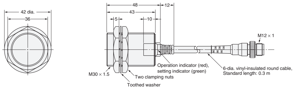
Fig. 35: E2E-X20MD1-M1GJ
