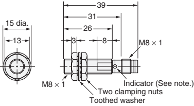
Fig. 28: E2E-X2D□-M3G/E2E-X1R5□-M3/F□-M3
