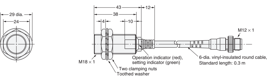
Fig. 32: E2E-X7D1-M1GJ E2E-X7D1-M1J-T
