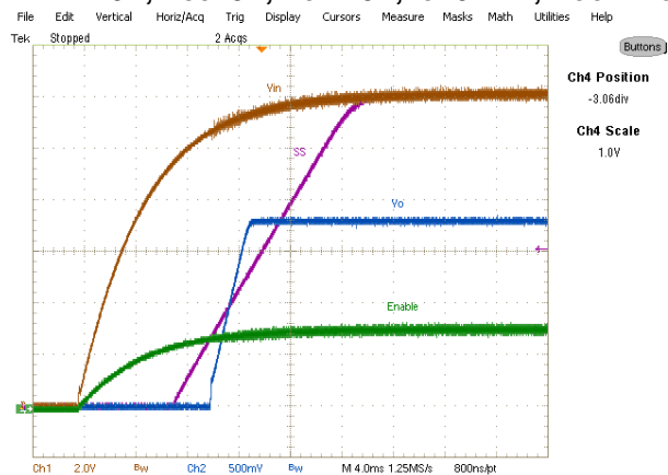
Fig. 7: Start up at 12A Load Ch 1 : V_{in} , Ch 2 : V_o , Ch 3 : V_{ss} , Ch 4 :Enable
