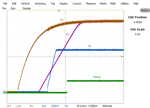
Fig. 8: Start up at 12A Load, Ch 1 : V_{in} , Ch 2 : V_o , Ch 3 : V_{ss} , Ch 4 : V_{PGood}
