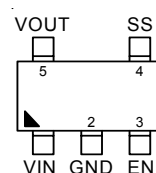
SOT-23-5 / SC-70-5
