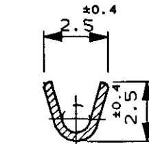
断面 A-A SECT A-A
