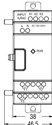
Expansion module
