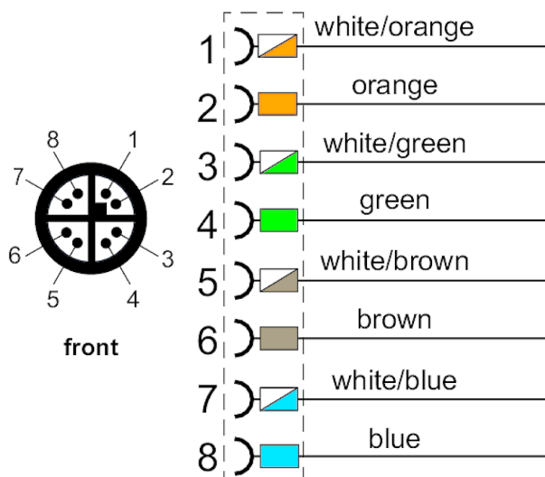
M12 jack
