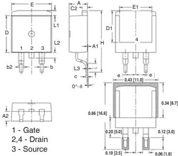
TO-263 Outline
