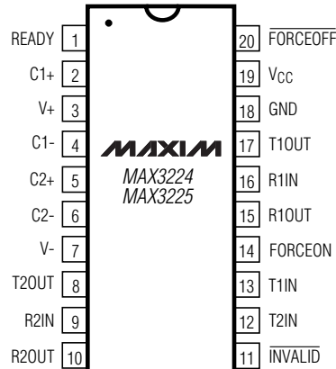
DIP/SSOP/TSSOP
