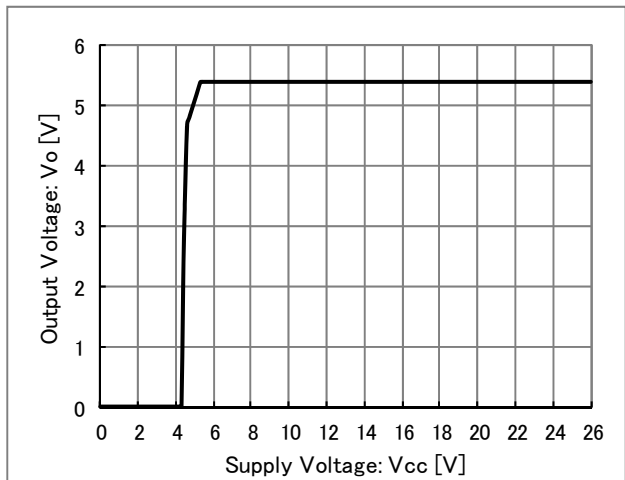
Figure 2. Vcc - Vo
