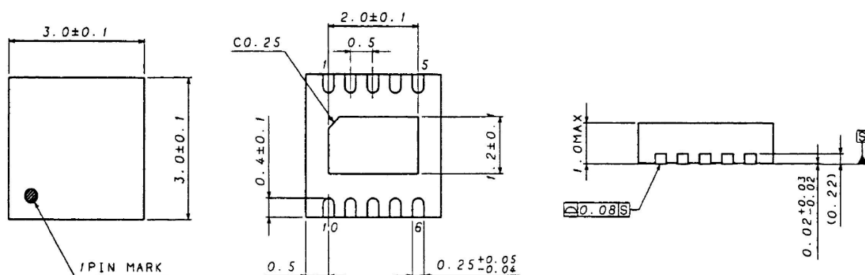
Package : VSON010V3030
