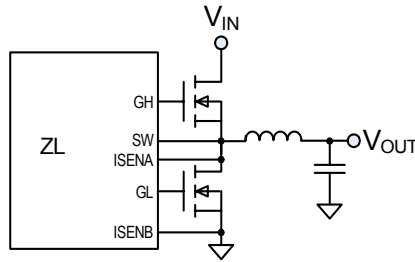
MOSFET R_{DS,ON} Sensing
