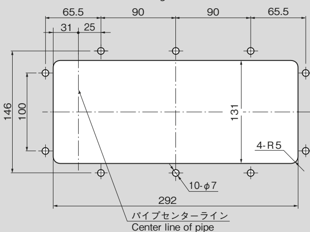
パネル穴明け寸法 Panel drilling dimensions
