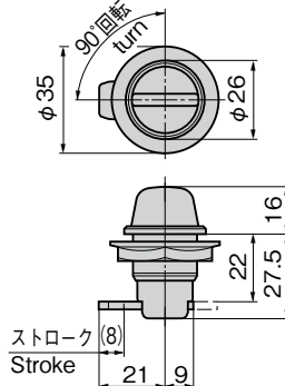
作動例(CP-315-A・AN) Example of operation
