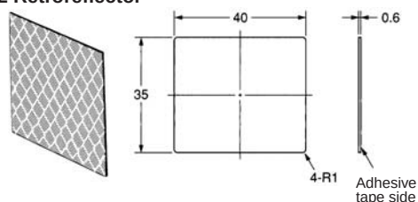
E39-RS2 Retroreflector
