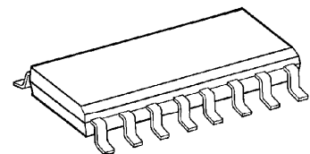
SOL16-P-150-1.27
