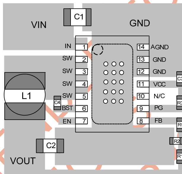
Top Layer
