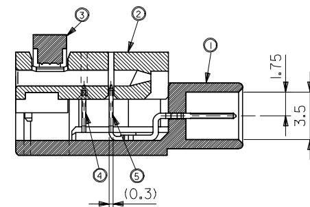
SECT A-A
