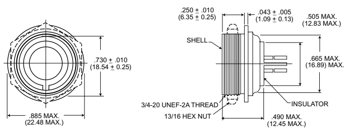
Receptacle
