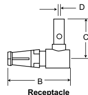
Receptacle
