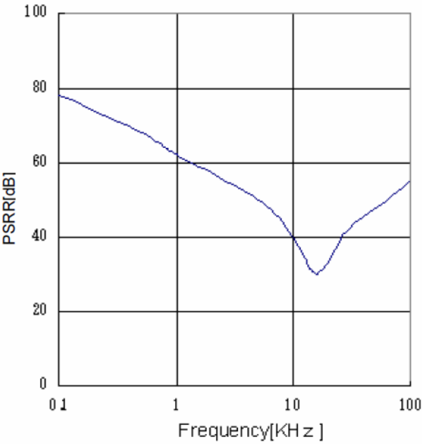
Fig. 32 PSRR (Io=0mA)
