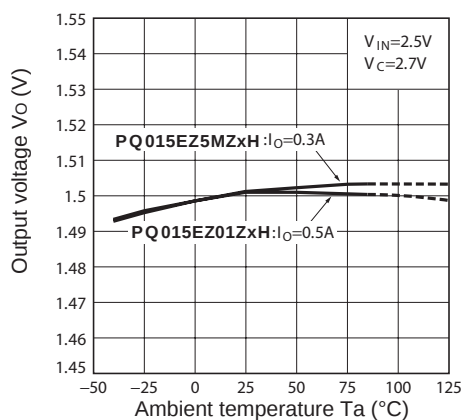
Fig.14 Output Voltage vs. Ambient Temperature (PQ015EZ5MZxH / PQ015EZ01ZxH)
