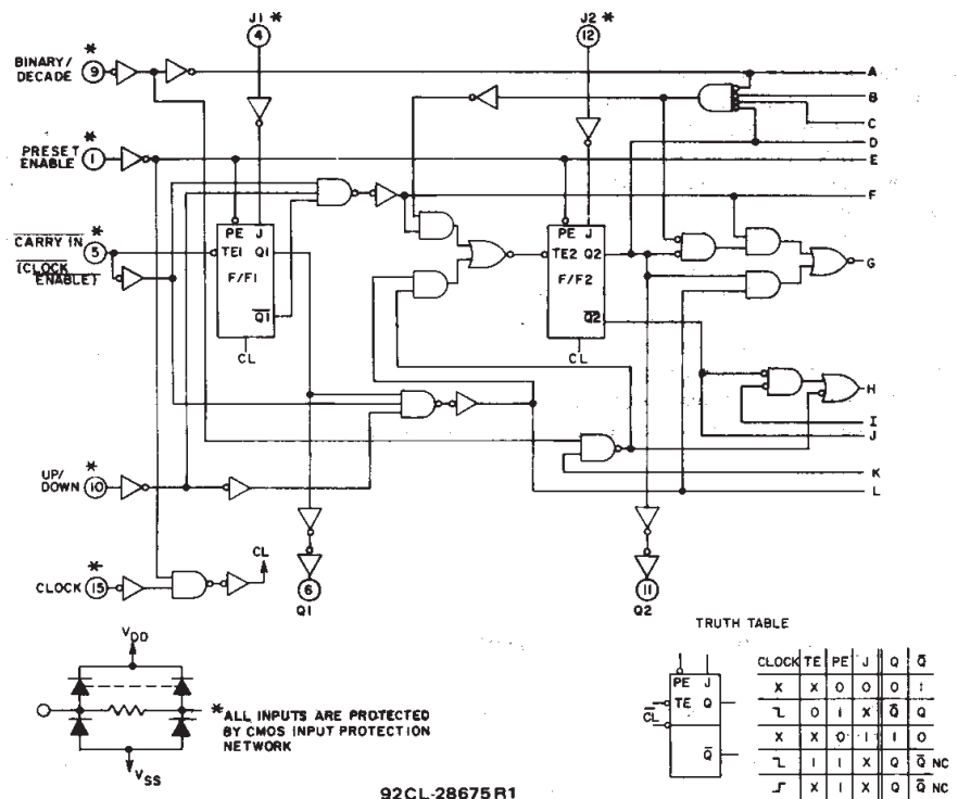
Fig. 9 - Logic diagram.
