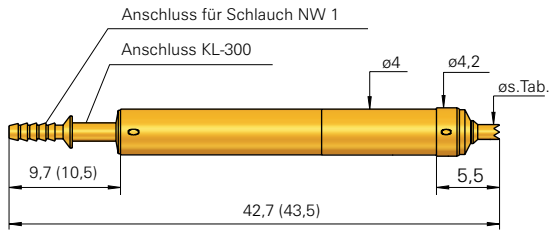
PKS-420 Typ 1: mit Anschluss für Schlauch NW 1
