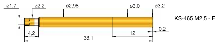
KS-465 M2,5 E05 - F
