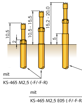
KS-465 M2,5 E05 - F - R (mit Rändel)
