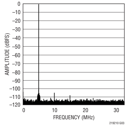
LTC2192: 64k Point FFT, f_{IN} = 5\text{MHz} , -1\text{dBFS} , 65\text{MSPS}
