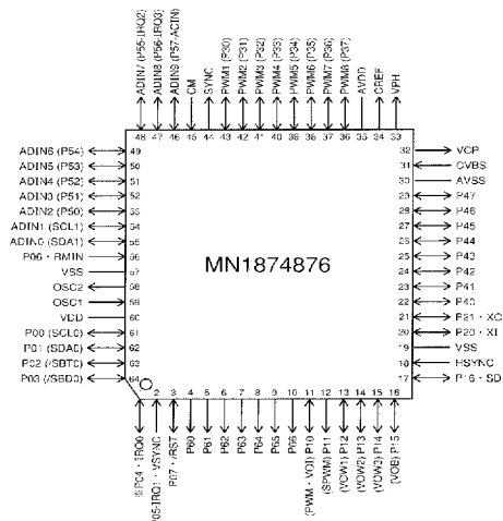
QFH064-P-1414B
