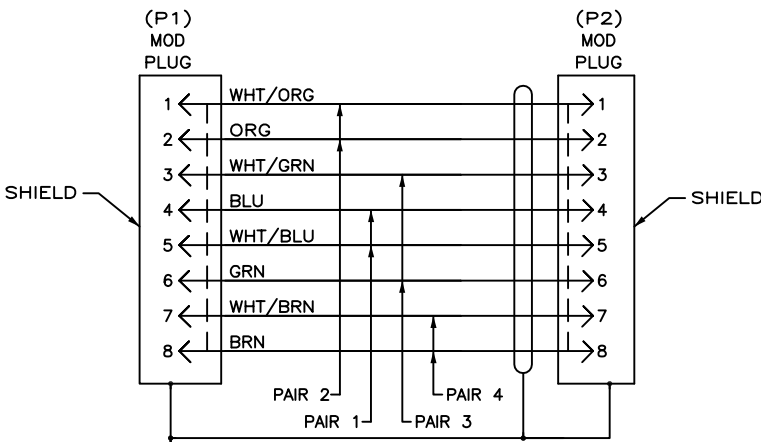
WIRING DIAGRAM 568B
