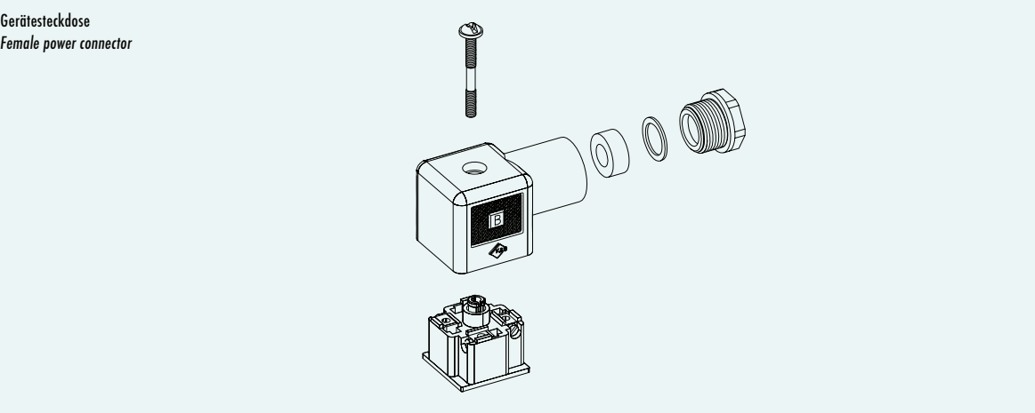
Gerätesteckdose mit Zugentlastung Female power connector with strain relief
