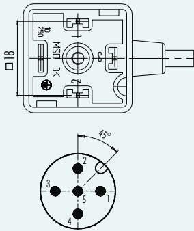
3+PE 3+PE
