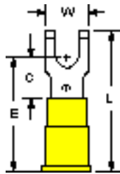
MVU10-8FFBK Stud Size 8 Wire Range 12-10
