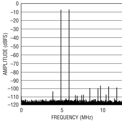
LTC2160: 64k Point 2-Tone FFT, f_{IN} = 69\text{MHz} , 70\text{MHz} , -7\text{dBFS} , 25\text{Mps}
