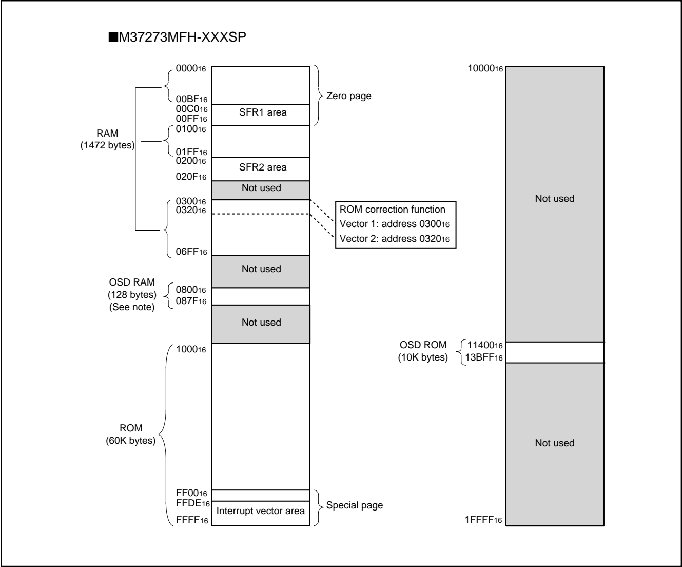
Fig. 8.2.1 Memory Map
