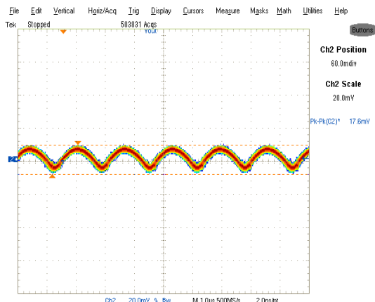
Fig. 20. Output Voltage Ripple, 2A load Ch_2: V_o
