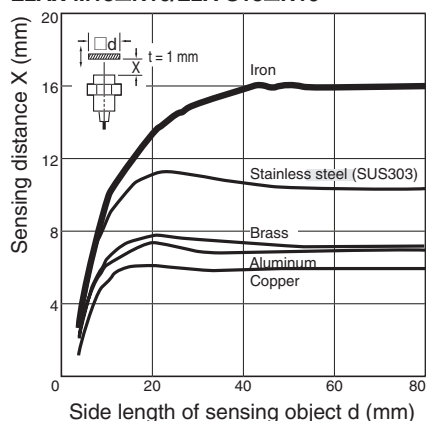
E2AX-M18□N16/E2A-S18□N16
