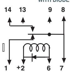
SPDT
