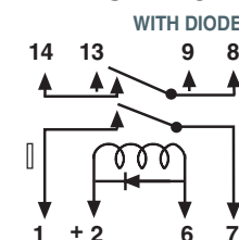
DPST - NO
