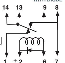
SPDT
