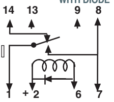
SPDT
